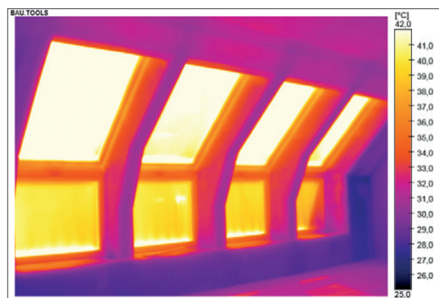
Endthermogramm: Unterschiede im Start- und Endthermogramm sind nicht erkennbar
